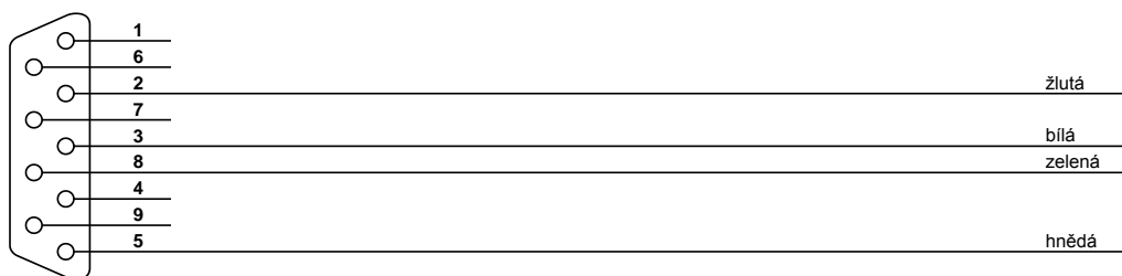
D-sub DE-9 vidlice
